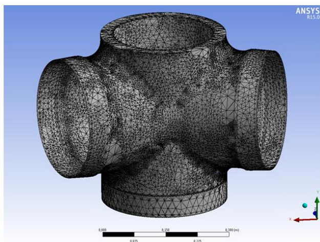
Рис. 2. Конечно-элементная модель поверхностного слоя траверсы
