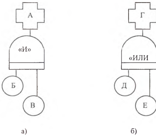
Рисунок 6.1 – Логические операции: а) – с логическим знаком «И», б) – с логическим знаком «ИЛИ»
