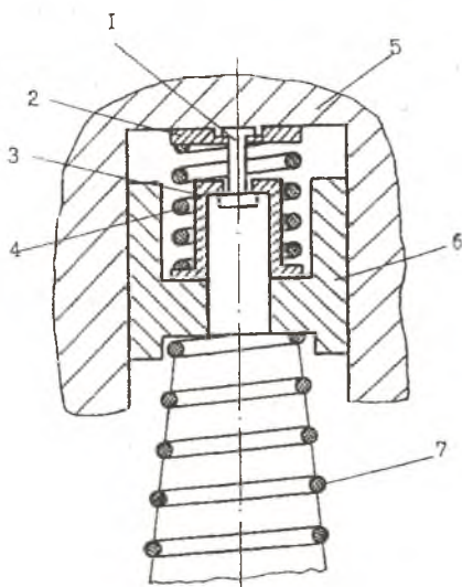
Р и с. 12. Узел центробежного регулятора с балансировочным пакетом: 1 - штифт; 2 - замковая шайба; 3 - втулка; 4 - пружина балансировочного пакета; 5 - корпус регулятора; 6 - зубчатая рейка; 7 - коническая пружина
