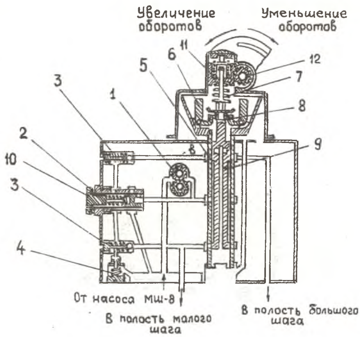
Р и с. 11. Схема устройства регулятора Р-9 СМ2: 1-маслонасоса; 2-редукционный клапан; 3-шариковый клапан; 4-перегрузочный клапан; 5-валик; 6-"Г"-образные грузики; 7-пружина; 8-шарикоподшипник; 9-золотник; 10-пробка; 11-зубчатая рейка; 12-шестерня валика ручного управления
