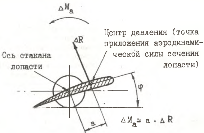
Р и с. 8. Схема образования момента от аэродинамических сил лопасти
