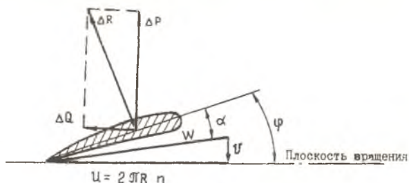
Р и с. 1. Треугольник скоростей и аэродинамические силы, действующие в сечении лопасти: u — окружная скорость; v — поступательная скорость (скорость полета); W — результирующая (истинная) скорость обтекания элемента лопасти
