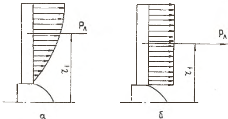
Р и с. 3. Эпюра элементарных сил тяги \Delta P по размаху лопасти: а - без геометрической кривки; б - с геометрической кривкой
