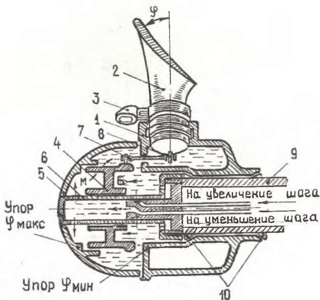
Р и с. 10. Схема устройства вента АВ-2: 1 - корпус; 2 - лопасть; 3 - противовес; 4 - поршень; 5 - цилиндр; 6 - труба маслопровода; 7 - шатун; 8 - палец стакана; 9 - носок вала вента; 10 - конусное кольцо
