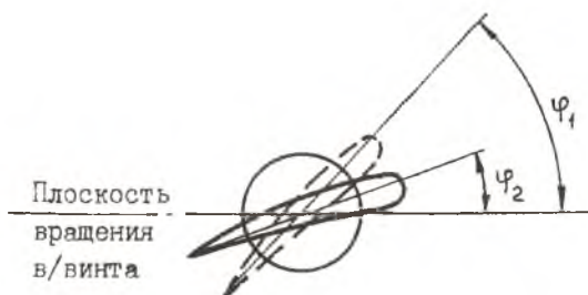
Р и с. 4. Схема расположения корневого и концевых сечений при геометрической кривке лопасти: \varphi_1 - угол установки корневого сечения; \varphi_2 - угол установки концевых сечения
