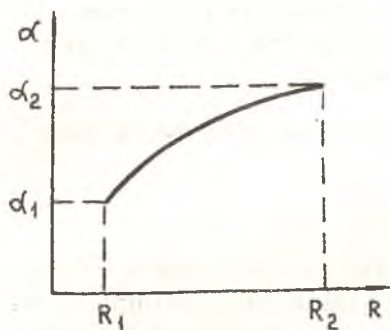
Р и с. 2. Характер изменения углов атаки \alpha сечений лопасти по радиусу в/винта R при постоянном по размаху угле установки: R_1 — корневое сечение лопасти; R_2 — концевое сечение лопасти
