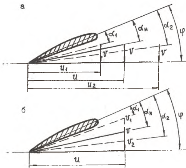
Р и с. 6. Зависимость углов атаки сечения лопасти от V и n при \varphi = \text{const} : а) V = \text{const} , n = \text{var} ; б) n = \text{const} , V = \text{var}
