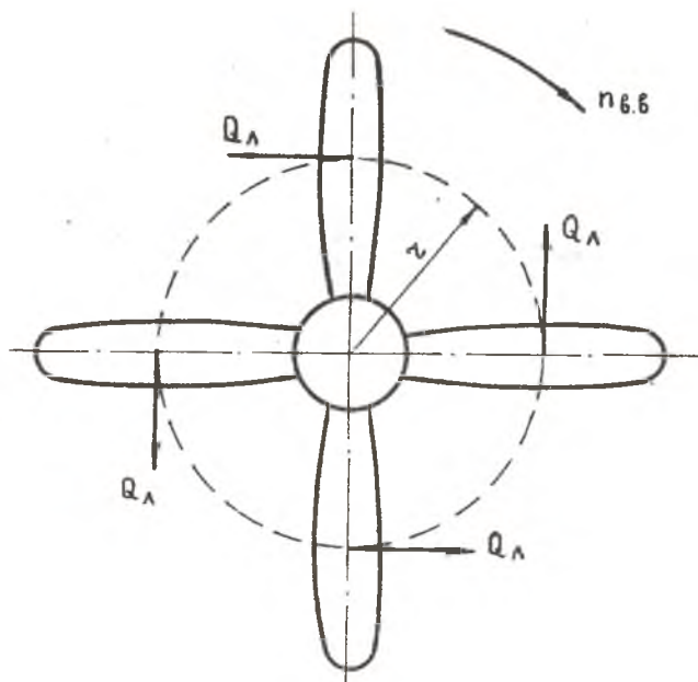
Р и с. 5. К определению момента сопротивления вращению в/винта
