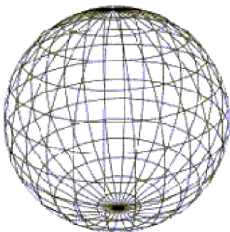
Рис. 3.1. Представление шара
