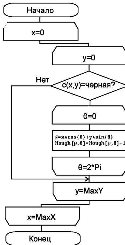
Рис. 2.38. Алгоритм Хафа
