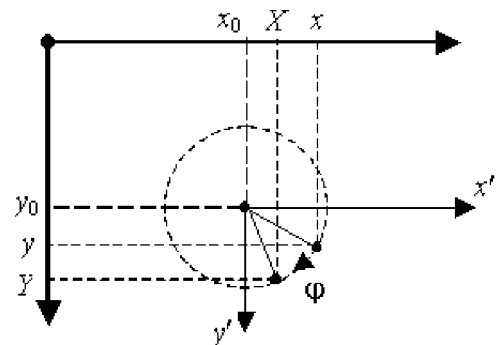
Рис. 2.18. Сложное преобразование
