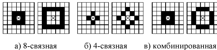
Рис. 2.31. Разновидности «волны»
