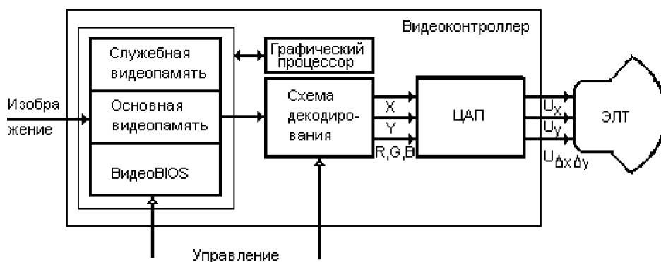
Рис. 1.34. Функциональная схема видеоподсистемы ПЭВМ
