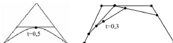
Рис. 2.1.2. «Геометрический» способ построения кривых Безье
