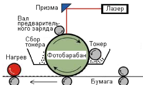
Рис. 1.29 Принцип действия лазерного принтера
