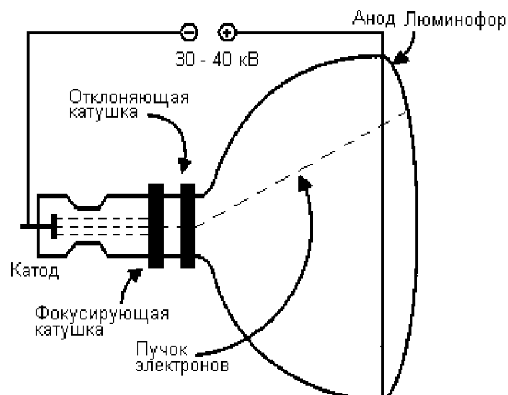
Рис. 1.26. Устройство электронно-лучевой трубки
