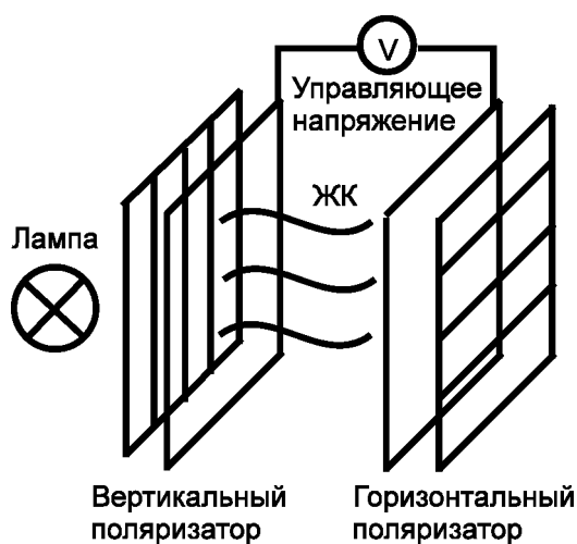
Рис. 1.27. Ячейка ЖК-матрицы
