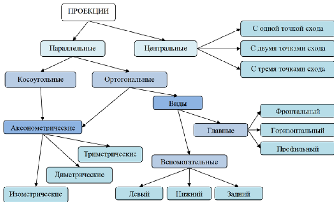
Рис. 2.20. Классификация проекций
