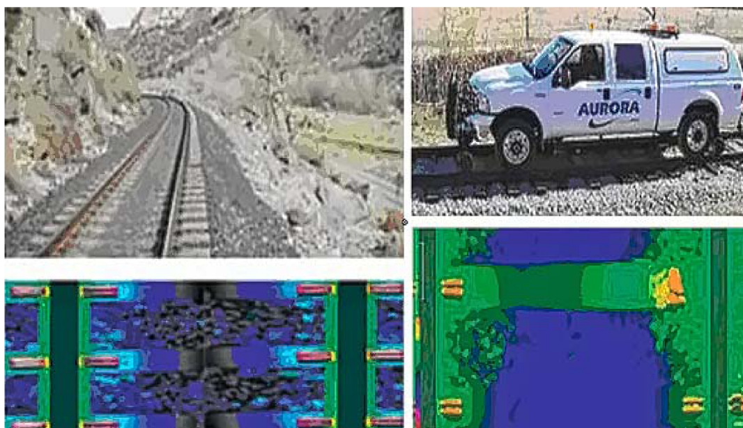
Рис. 1.3. 3D-камера фиксирует сломанную шпалу на скорости 50 км/ч
