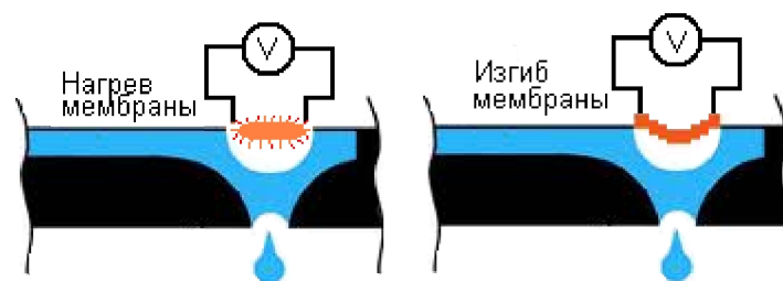
Рис. 1.28. Принципы действия струйных принтеров
