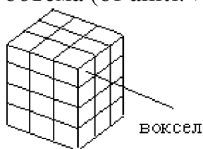
Рис. 3.3. Трехмерный растр
