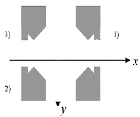
Рис. 2.17. Отражения объекта
