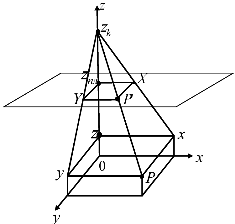
Рис. 2.23. Перспективное проектирование
