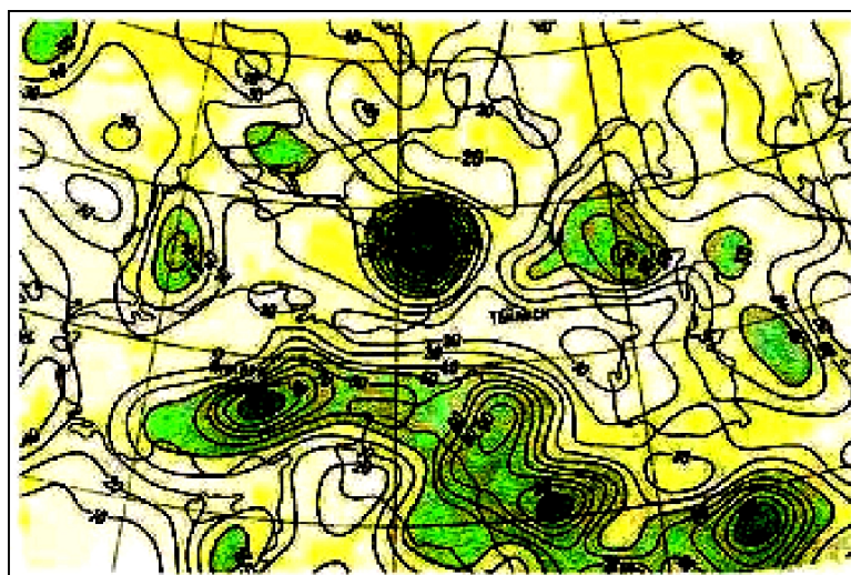
Рис. 3.6. Изолинии
