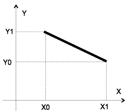
Рис. 2.1. Отрезок прямой
