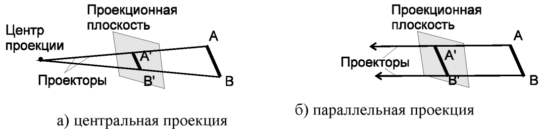
Рис. 2.19. Виды проекций
