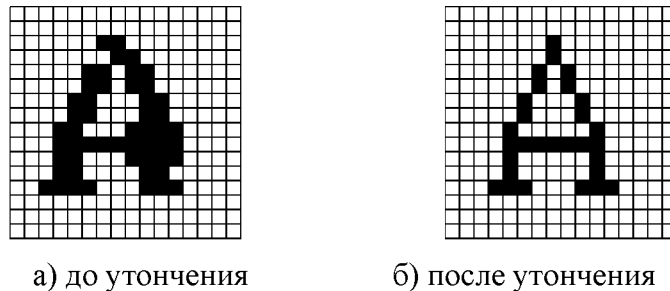
Рис. 2.29. Утончение линий
