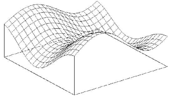
Рис. 3.5. Равномерная сетка
