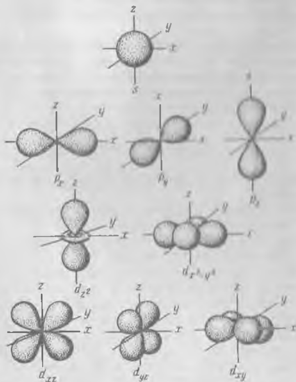
Р и с. 1. Формы s -, p - и d -электронных облаков (орбиталей)
