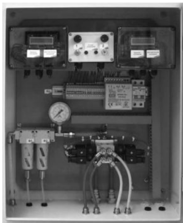
Рисунок 3 - Шкаф серии BOH для дистанционного управления электропневматическими позиционными и следящими приводами
