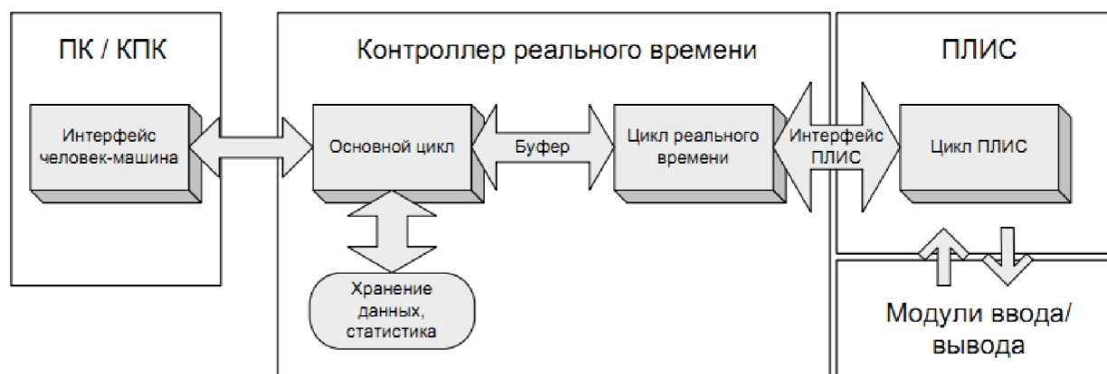
Рис. 3 Программная архитектура подсистемы
