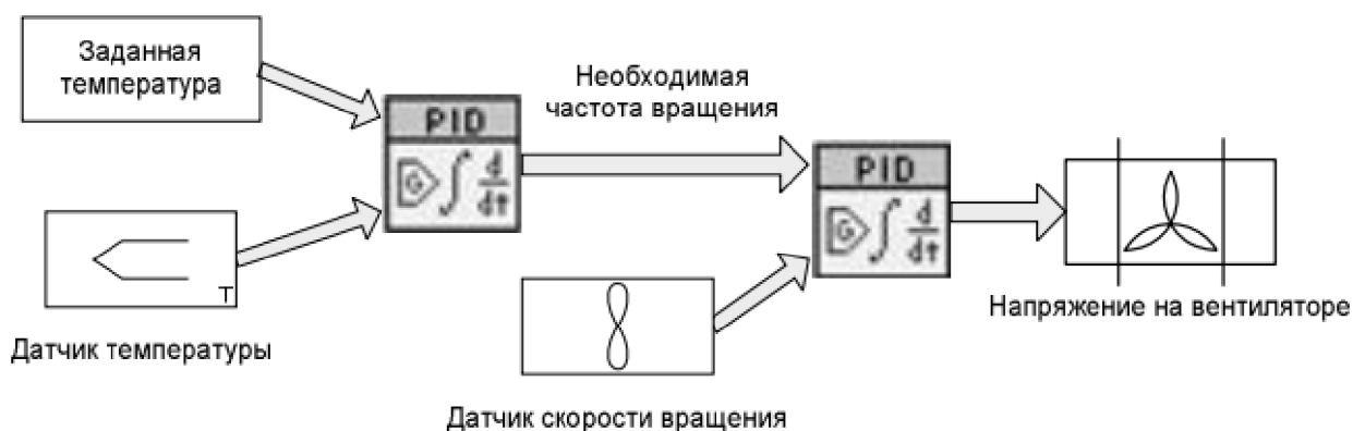
Рис. 4 Схема управляющего алгоритма
