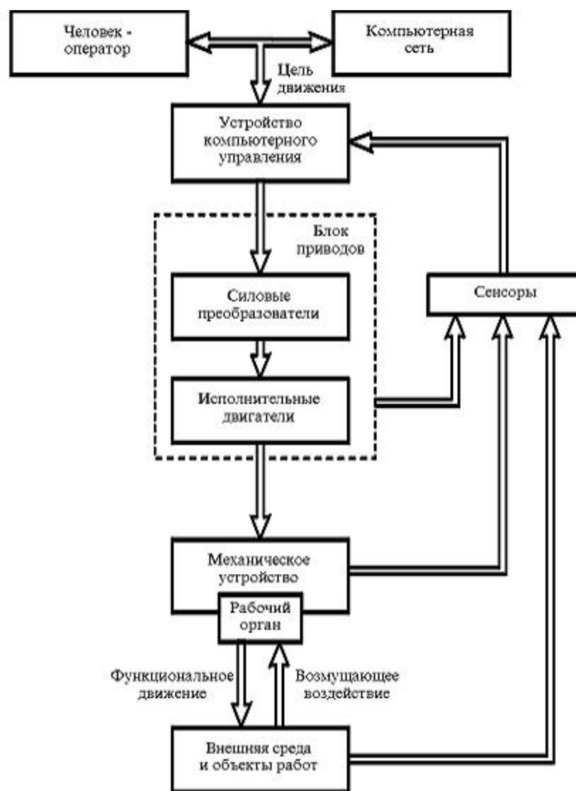
Рисунок 1 - Обобщенная схема машины с компьютерным управлением движением
