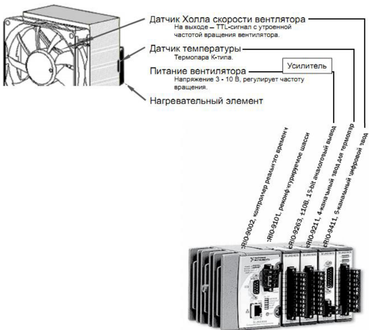
Рис. 1 Схема установки
