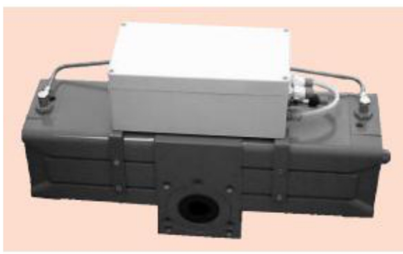
Рис. 5. Электропневматический позиционный привод на базе поворотного пневмоцилиндра
