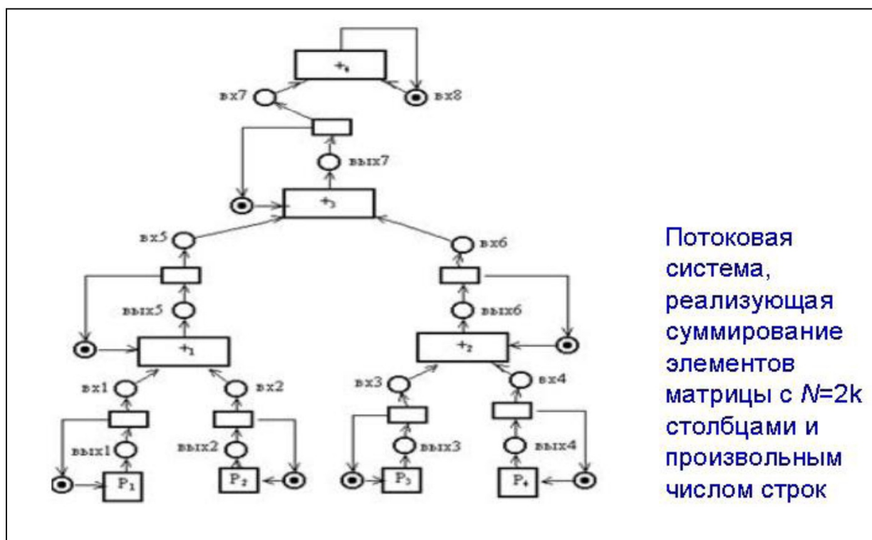
Рис. 1.7. Пример Сети Петри
