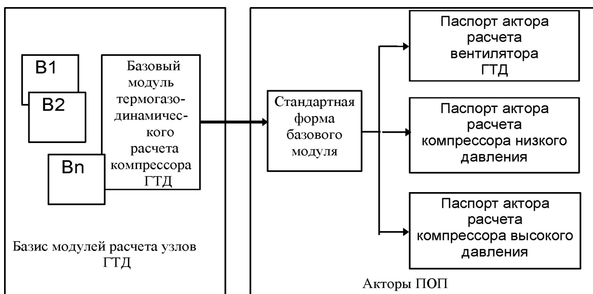
Рис. 2.1. Порождение акторов в предметной области
