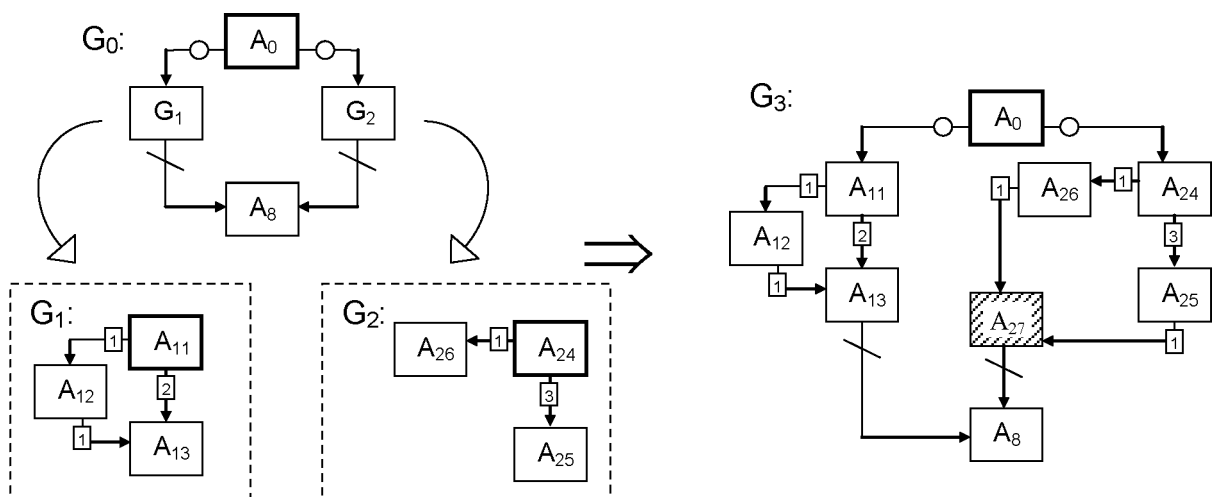
Рис. 5.3 – Исключение иерархии из модели вычислительного процесса
