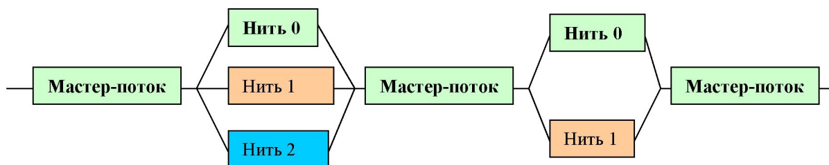
Рисунок 4.3 – Модель «пульсирующего» параллелизма технологии OpenMP
