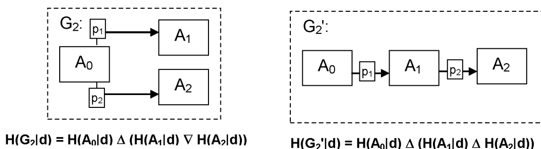
Рис. 5.5 – Замена операции ветвления на операцию следования
