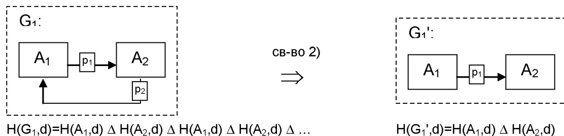
Рис. 5.8. Исключение циклических участков модели при построении формул над способами использования данных
