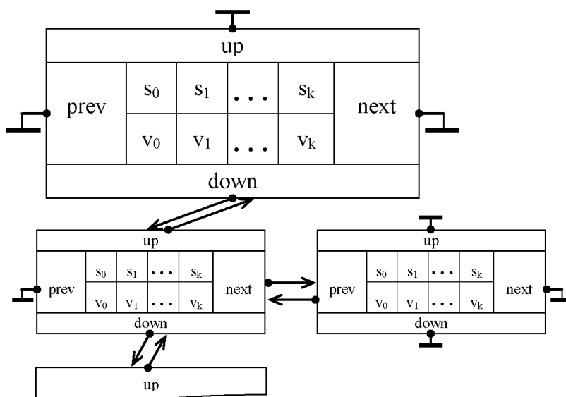
Рис. 5.23. Представление покрывающего дерева в памяти ЭВМ
