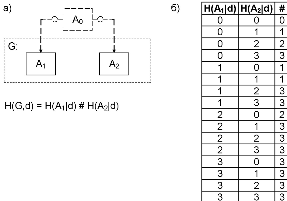
Рис. 5.6 – Операция параллельного исполнения
