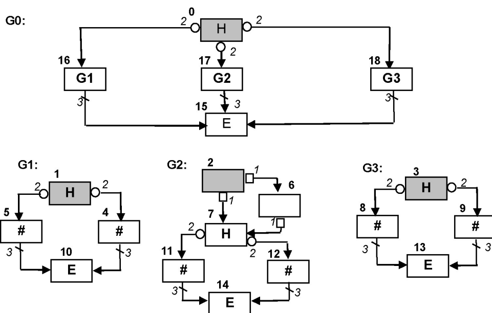
Рис.4.7. Разбиение агрегата G0 на правильные
