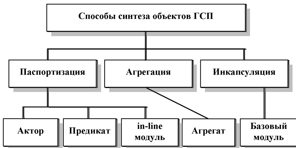
Рис 3.1. Способы синтеза объектов ГСП
