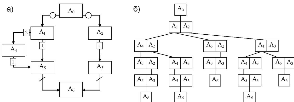
Рис. 5.22. Пример покрывающего дерева, соответствующего граф-модели параллельного вычислительного процесса
