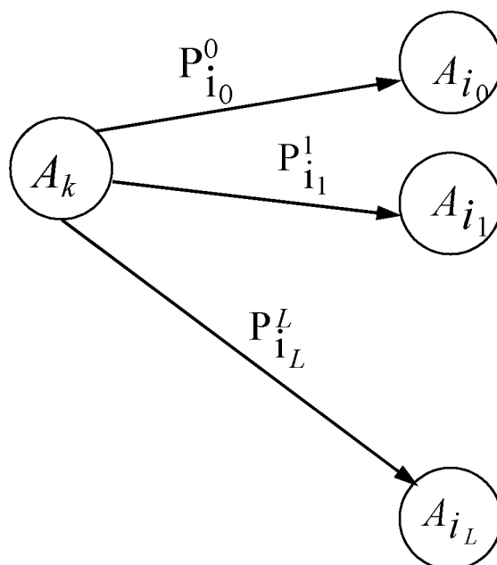
Рис. 2.6 Фрагмент граф-программы
