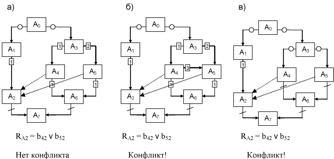
Рисунок 4.2 – Пример использования операции "v" в семафорных предикатах
