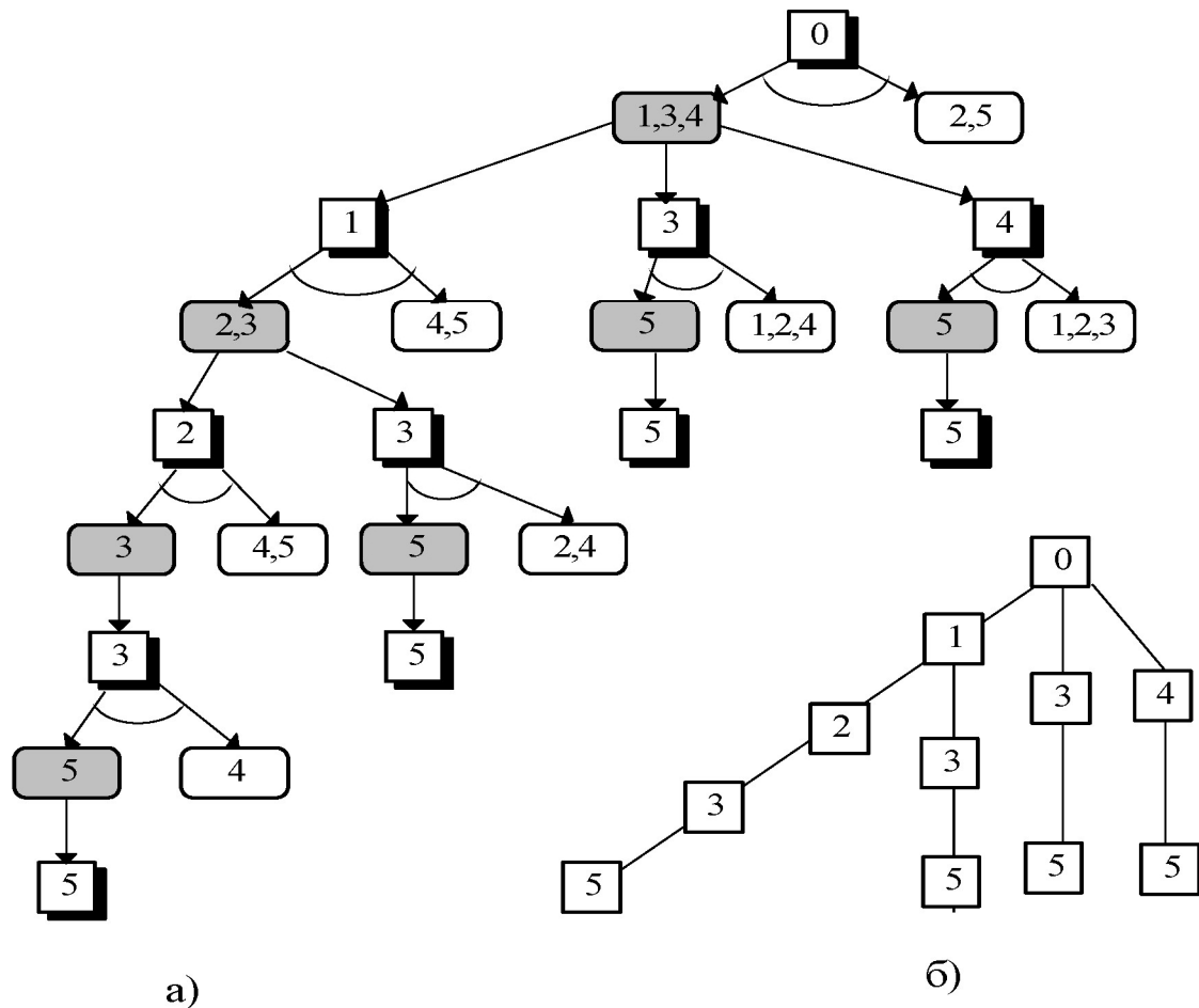
Рис.3.10. И/ИЛИ-граф алгоритма АЧП
