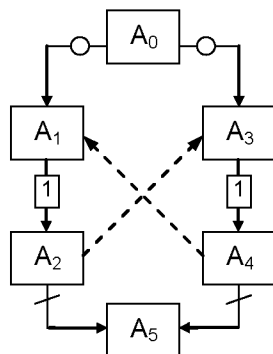
Рис. 5.21. Пример граф-модели, содержащей тупик
