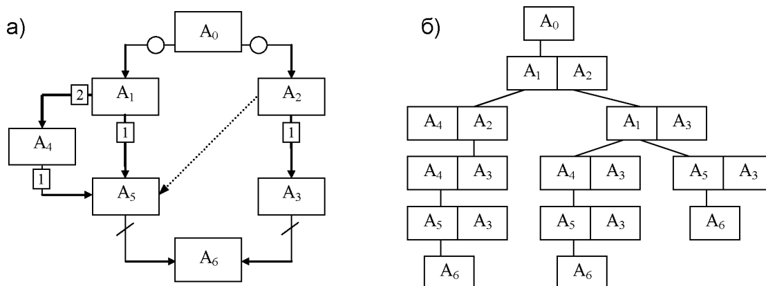
Рис. 5.25. Синхронизация вершин, совместно использующих данные
