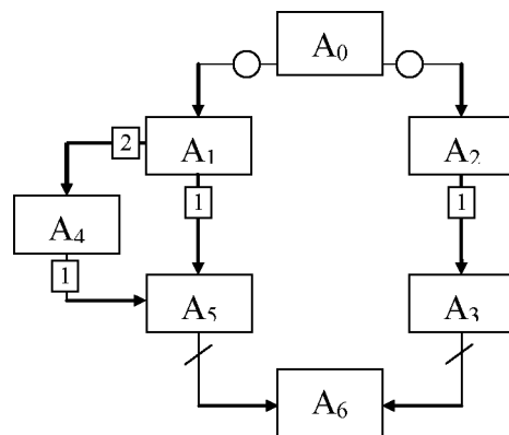
Рис. 5.24. Пример модели параллельных вычислений
