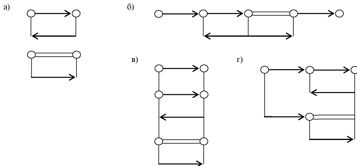
Рис. 1.8. Пример построения Р-схем
