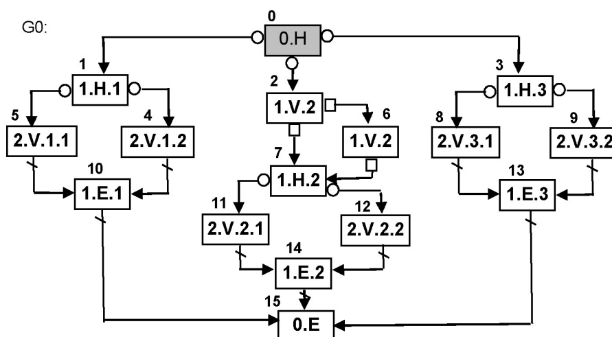
Рис. 4.8. Размеченный граф
