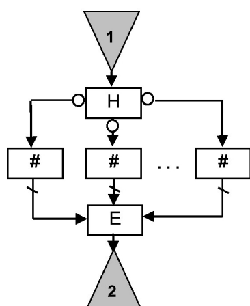
Рис 4.5. Правильно построенный агрегат
