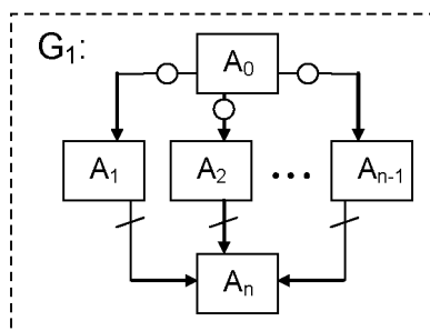
Рисунок 5.9 – Элементарная параллельная граф-модель
