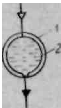
Рис. 2.11. Вытеснение компонентов из бака в невесомости
