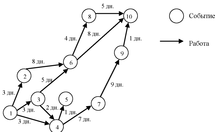
Рис. 3.2. Пример упрощенной сети
