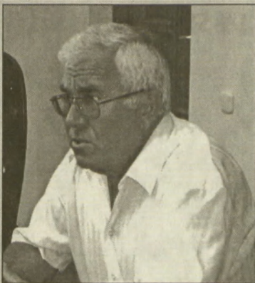
Координатор работ российских институтов по международному проекту Большой адронный коллайдер в ЦЕРНе (Швейцария), замдиректора Научно-исследовательского института ядерной физики МГУ (НИИ ЯФ МГУ) по научной работе, профессор Виктор Иванович Саврин; замдиректора Санкт-Петербургского института ядерной физики Российской Академии Наук (ПИ ЯФ РАН) по научной работе, профессор Владимир Михайлович Самсонов; директор отделения нейтронных исследований ПИ ЯФ РАН, профессор Валерий Васильевич Федоров; ректор Самарского Госуниверситета, профессор Геннадий Петрович Яровой.
