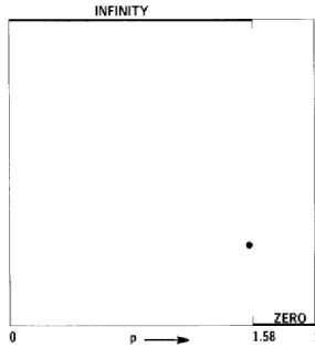
Рис.21. Размерность меры – скачкообразное поведение (Barnsley M. F. Fractals Everywhere . AP, 1988)
