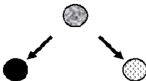
Рис. 1. Антиномия материи
