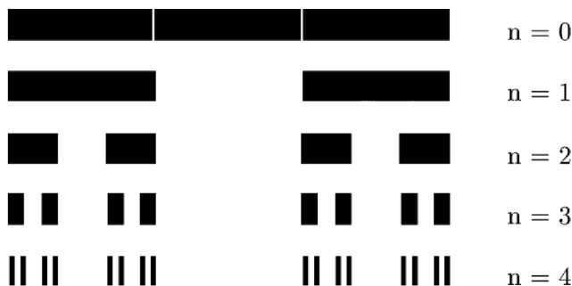
Рис. 16. Канторово совершенное множество C
