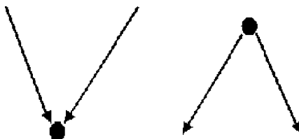
Рис. 5. Конвергенция – дивергенция
