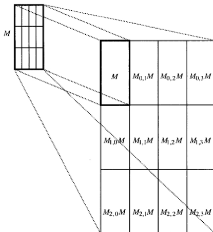
Рис. 29. Фракталы и Матрицы
