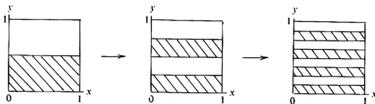
Рис. 15. Преобразование пекаря
