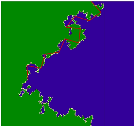
Рис. 8. Типичная береговая линия
