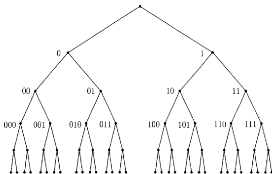
Рис. 27. Дерево 2-адических чисел p = 2 . (Badii R., Politi A. Complexity . CUP, 1997.)
