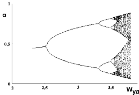
Рис. 12. Удвоение периода. Логистическое уравнение
