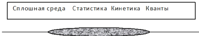
Рис. 19. Материя в диапазоне размеров
