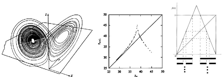
Рис. 14 Отображение «треугольник»
