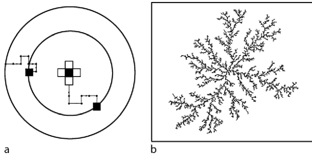
Рис. 18. Образование DLA кластера
