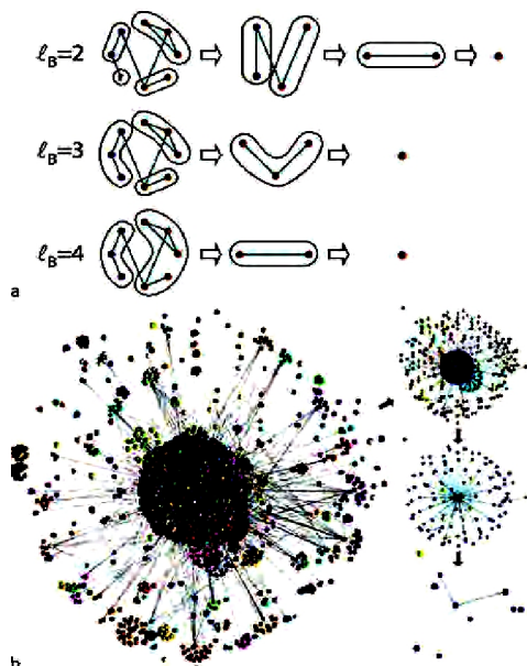
Рис. 10. Масштабно инвариантная сеть. Образование кластеров (Meyers R.A. Encyclopedia of Complexity and Systems Science . Springer, 2010)
