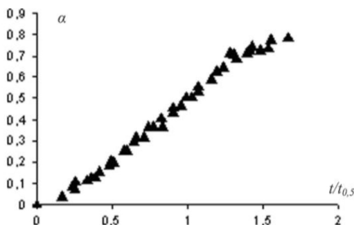
Рис. П1.1. Зависимость доли растворенного оксида \alpha от приведенного времени на примере никеля (II) и оксида никеля (III)
