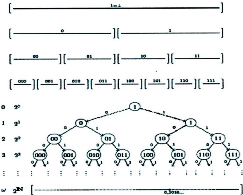
Рис. 24. Образование канторовой пыли совместно с бинарным лексикографическим деревом. Итеративная система функций (Verelst K. Zeno's Paradoxes .// arXiv:0606639v1 [math.HO] 2006)
