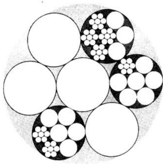
Рис. 28. Строеие множества Z_7 (Schilhoff W. H. Ultrametric Calculus . CUP, 1984)
