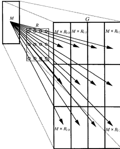
Макроскопический вид матрицы G = M \otimes R .
