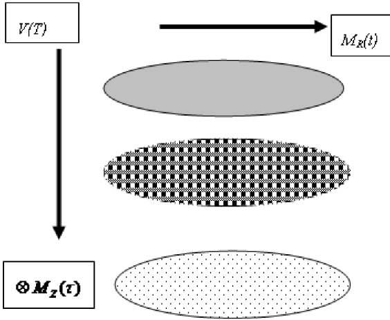
Рис. 30. Двумерная семантика модели
