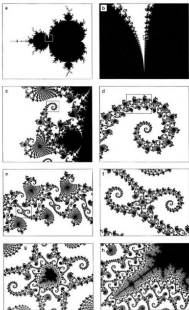
Рис. 11. Множество Мандельброта на нескольких масштабах
