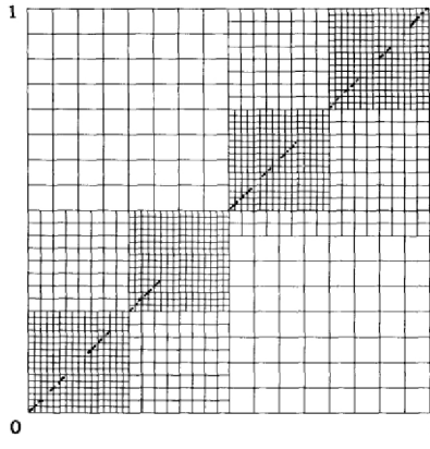
Рис. 22. Процедура измерения фрактальной размерности канторова множества C (диагональ квадрата). Уплотняющаяся сетка покрывающих эталонов представлена вложенными квадратами (Barnsley M.F. Fractals Everywhere . Ac.Press, 1988)
