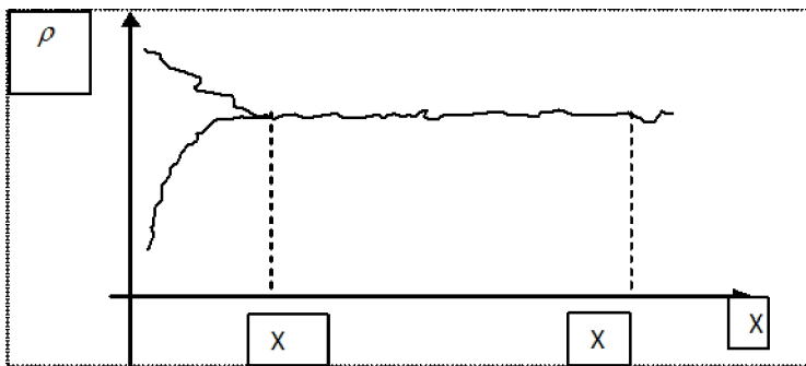
Рис. 6. Промежуточная асимптотика
