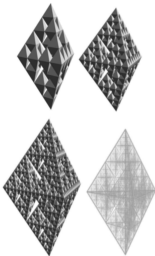
Рис.2. Антиномия материи (продолжение) (Lipscomb S. Fractals and Universal Sets in Dimension Theory . Springer 2009, Ch.2.)
