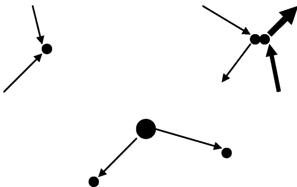
Рис. 7. Траектории частиц. Динамическая природа фрактальной геометрии
