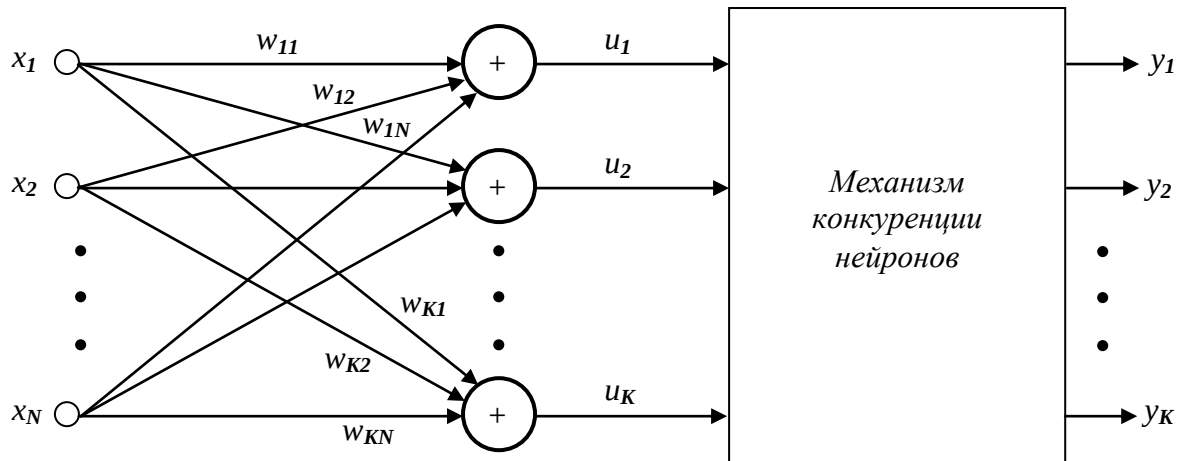
Рис. 1.8 Схема соединения нейронов типа WTA
