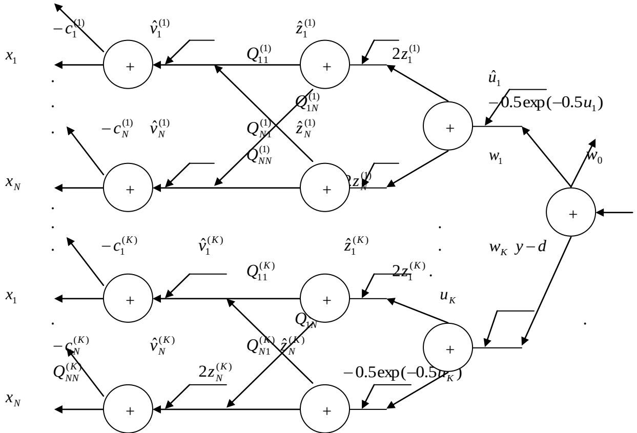
Рис. 3.5. Структура сопряженной HRBF-сети, используемая для расчета градиента
