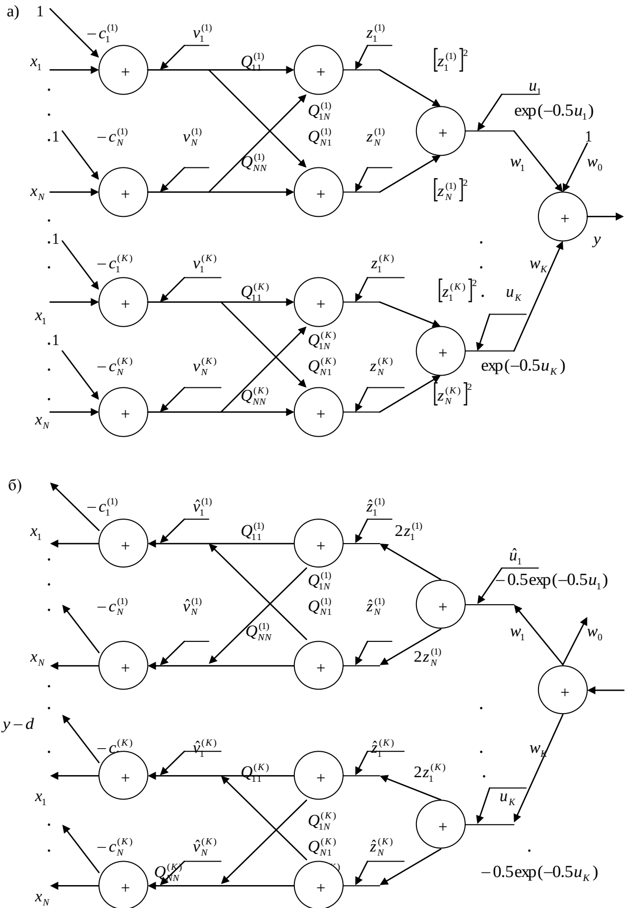
Рис. 3.4. Структура HRBF-сети, используемая для расчета градиента
