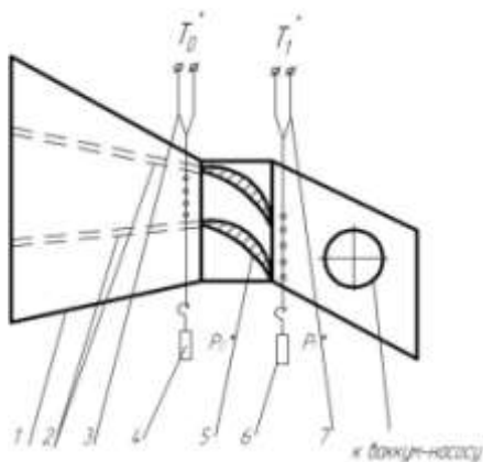
Рис. 1.5. Схема препарирования стэнда для экспериментального исследования плоских решеток
