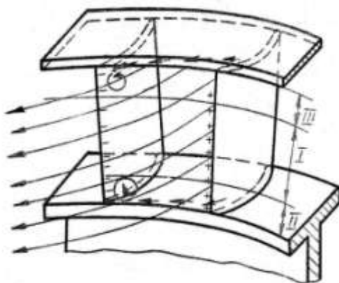
Рис. 1.1. Схема течения потока в лопаточном венце турбомашины
