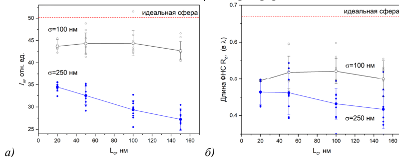
Рис. 3. Зависимость пиковой интенсивности ФНС I_m (а) и протяженности R_z (б) от длины корреляции искажений поверхности микросферы L_c
