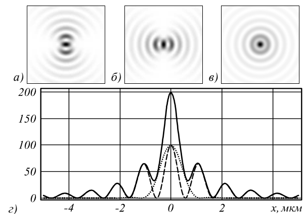
Рис. 3. Результаты моделирования формирования вихревого пучка Бесселя с азимутальной поляризацией, показана интенсивность центральной части компонент электрического поля: x-компонента (а), y-компонента (б), а также полная интенсивность (в) и соответствующие сечения (г) (x-компонента – точечная линия, y-компонента – пунктирная линия, полная интенсивность – сплошная линия)
