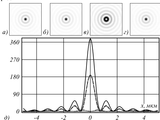
Рис. 1. Результаты моделирования формирования пучка Бесселя нулевого порядка с круговой поляризацией, показана интенсивность центральной части компонент электрического поля: x -компонента (а), y -компонента (б), z -компонента (в), а также полная интенсивность (г) и соответствующие сечения (д) ( x -компонента – точечная линия, y -компонента – пунктирная линия, z -компонента – штрихпунктирная линия, полная интенсивность – сплошная линия)
