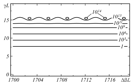
Рис. 3. Контуры равных коэффициентов усиления обратной TE-моды ( n = 0 ) на плоскости \Delta\beta L - \gamma L ; длина волны \lambda = 10,6 мкм, толщина плёнки t_{WG} = 10 мкм, длина резонатора L = 0,1 см, коэффициент связи \kappa_{00} \approx 0,007 \text{ см}^{-1}
