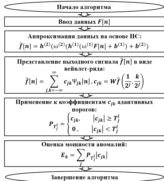
Рис. 1. Блок-схема алгоритма анализа данных сложной структуры
