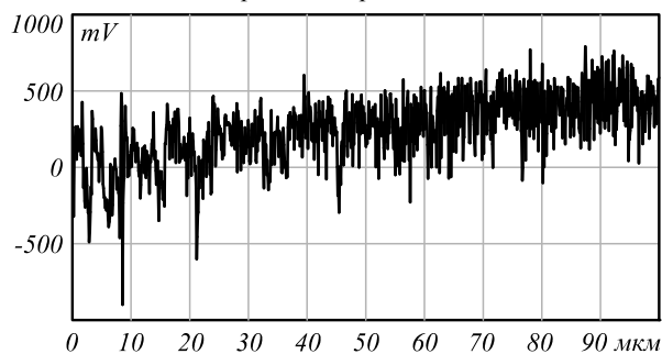
Рис. 2. Действие латеральных сил на отклонение от нормали кантилевера (образец №1) при сканировании в обратном направлении
