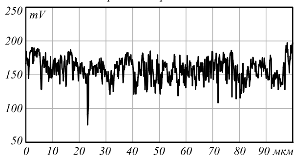
Рис. 4. Действие латеральных сил на отклонение от нормали кантилевера (образец №2) при сканировании в обратном направлении
