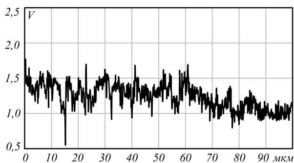
Рис. 1. Действие латеральных сил на отклонение от нормали кантилевера (образец №1) при сканировании в прямом направлении
