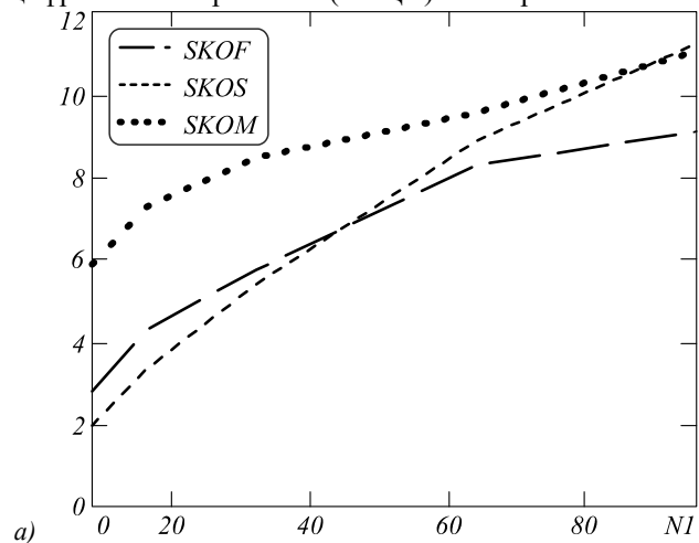
Рис. 7. SKO, вычисленные для фрагментов рис. 6а, б соответственно: SKOF (МИПВС – прерывистая линия), SKOS (сплайн – пунктир), SKOM (нейронная сеть – полужирный) в зависимости от NI (ширина нижней части моделируемой лакуны)
