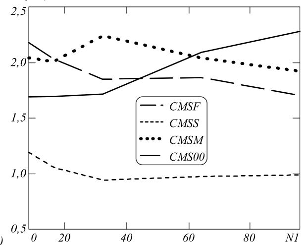
Рис. 9. МРЦИ, вычисленные для фрагментов рис. 6а, б соответственно: CMSF (МИПВС – прерывистая линия), CMSS (сплайн – пунктир), CMSM (нейронная сеть – полужирный), CMS00 (исходные неискажённые данные – сплошная линия) в зависимости от NI (ширина нижней части моделируемой лакуны)
