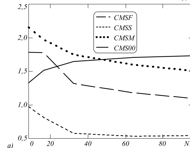
Рис. 9. МРЦИ, вычисленные для фрагментов рис. 6а, б соответственно: CMSF (МИПВС – прерывистая линия), CMSS (сплайн – пунктир), CMSM (нейронная сеть – полужирный), CMS00 (исходные неискажённые данные – сплошная линия) в зависимости от NI (ширина нижней части моделируемой лакуны)
