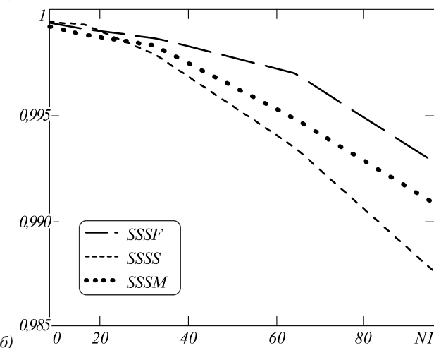
Рис. 8. MCP, вычисленные для фрагментов рис. 6а, б соответственно: SSSF (МИПВС – прерывистая линия), SSSS (сплайн – пунктир), SSSM (нейронная сеть – полужирный) в зависимости от NI (ширина нижней части моделируемой лакуны)
