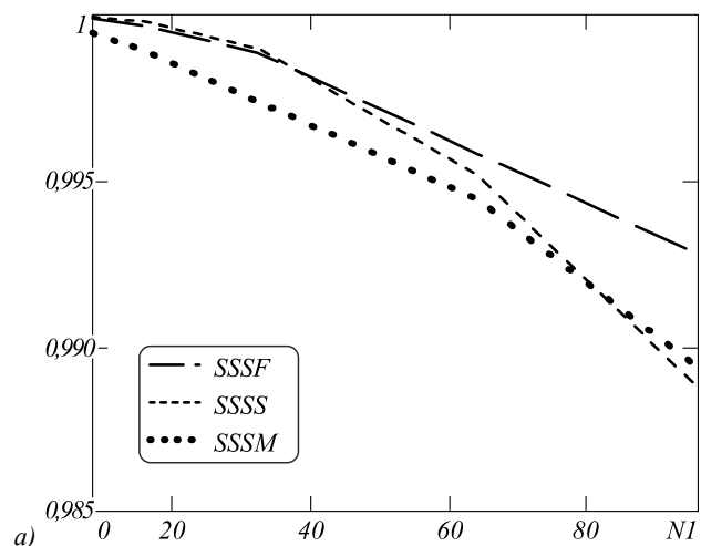
Рис. 8. MCP, вычисленные для фрагментов рис. 6а, б соответственно: SSSF (МИПВС – прерывистая линия), SSSS (сплайн – пунктир), SSSM (нейронная сеть – полужирный) в зависимости от NI (ширина нижней части моделируемой лакуны)
