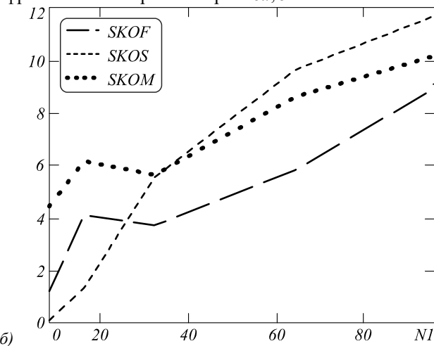
Рис. 7. SKO, вычисленные для фрагментов рис. 6а, б соответственно: SKOF (МИПВС – прерывистая линия), SKOS (сплайн – пунктир), SKOM (нейронная сеть – полужирный) в зависимости от NI (ширина нижней части моделируемой лакуны)
