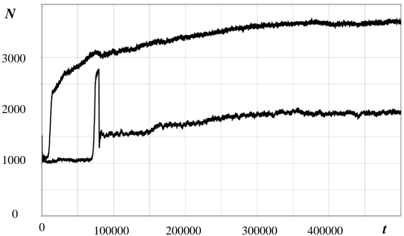
Рис. 1. Зависимость численности популяции N от времени t в полной модели (нижняя кривая) и в случае «глобального пацифизма» (верхняя кривая).
