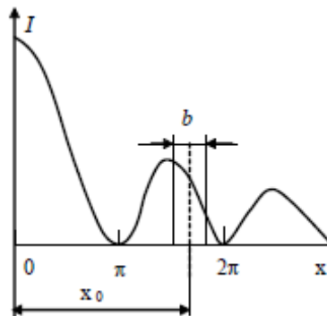
Рис. 3.9. Схема расчета влияния полевой диафрагмы
