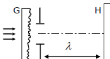
Рис. 8.20. Схема регистрации спекл-картины на фотопластинке Н
