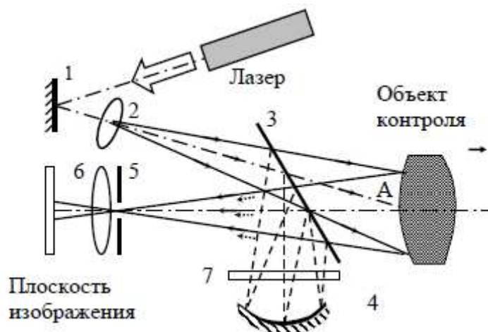
Рис. 8.29. Схема спекл-интерферометра. 1-поворотное зеркало; 2- микрообъектив; 3- светоделительная пластинка; 4-сферическое зеркало; 5- регулируемая диафрагма; 6- объектив CCD; 7-поляризационный светофильтр
