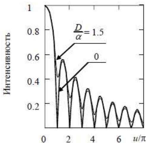
Рис. 6.10. Влияние пространственной когерентности излучения на ДК
