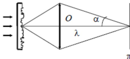
Рис. 8.10. Размер субъективного спектра
