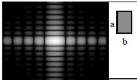
Рис. 2.6. Фурье-преобразование от прямоугольного отверстия.
