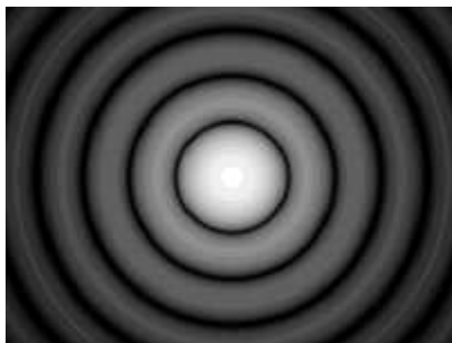
Рис. 2.7. Фурье-преобразование от круглого отверстия.
