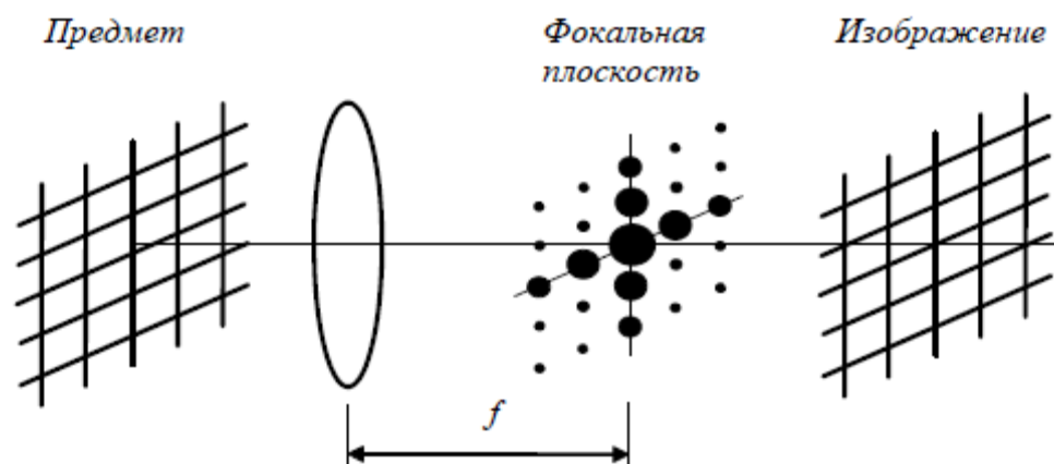
Рис. 3.4. Схема эксперимента Аббе-Портера
