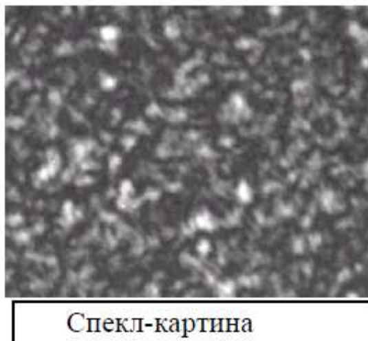
Рис. 8.1. Спекл-картина, получаемая при освещении лазером сильно шероховатой поверхности
