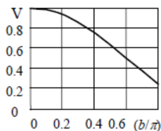
Рис. 3.10. Влияние ширины щели фотоприемника на контраст ДК
