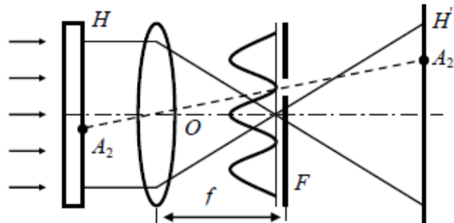
Рис. 8.24. Выявление в плоскости Н' разницы двух изображений
