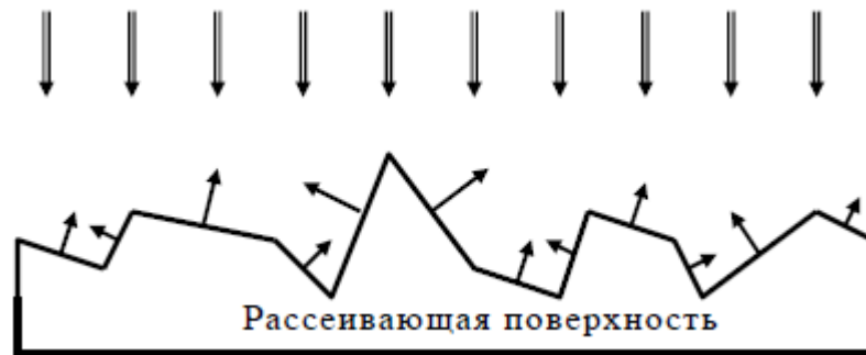
Рис. 8.2. Модель рассеяния на шероховатой поверхности
