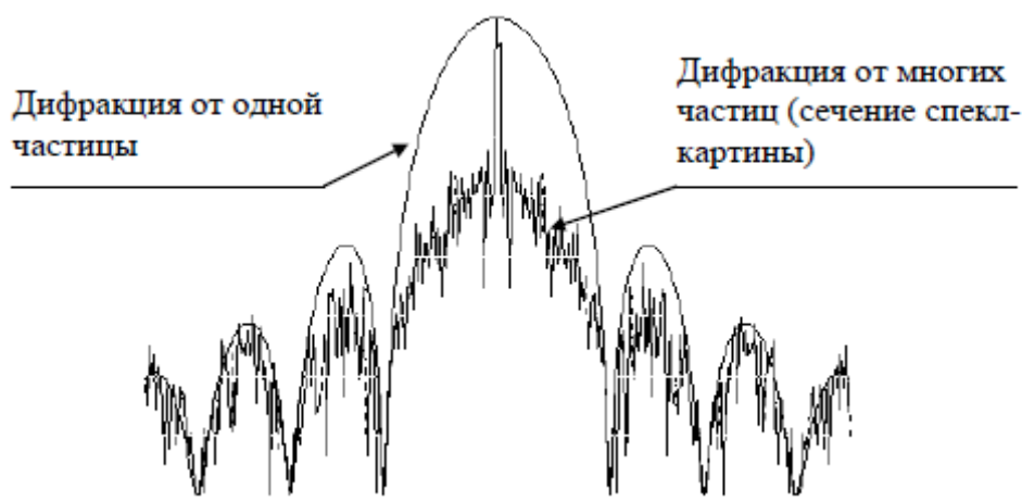
Рис. 8.8. Сечение дифракционной картины при дифракции на одной и на множестве одинаковых частиц Дифракция от многих частиц
