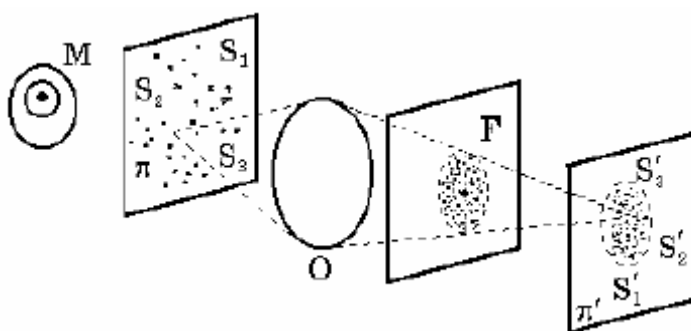
Рис. 8.7. Изображение большого числа хаотически расположенных источников
