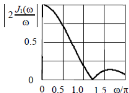
Рис. 4.2. Функция когерентности для источника круглой формы единичного радиуса
