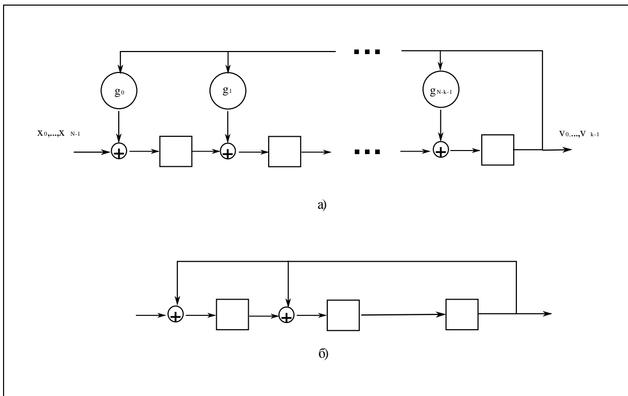
Рисунок 22.2. Реализация деления полиномов с помощью регистров сдвига.
