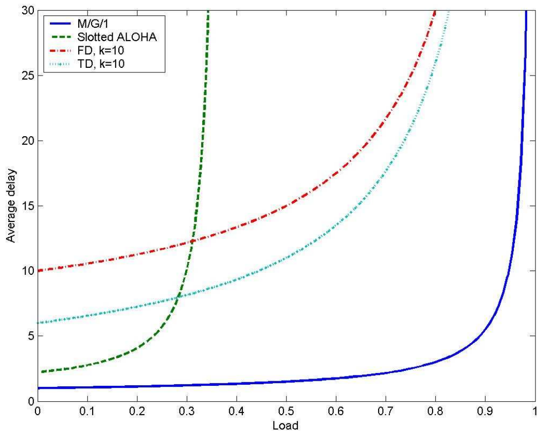
Рисунок 31.1. Задержки различных методов разделения канала.
