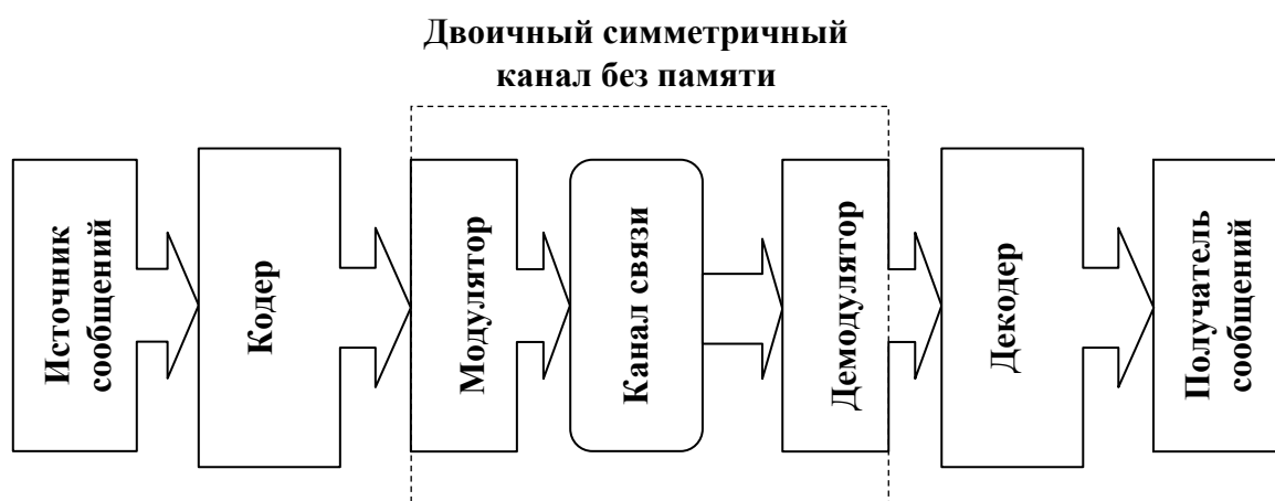
Рисунок 18.1. Система связи с каналом передачи символов
