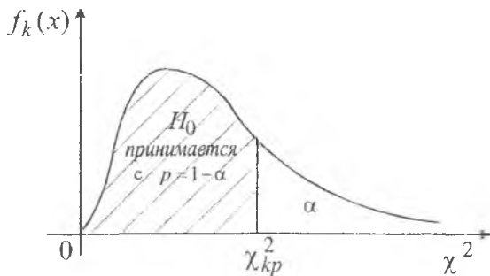
Р и с. 10. Область принятия гипотезы в критерии согласия
