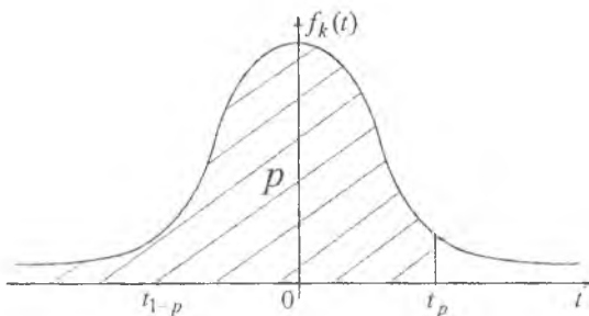
Р и с. 9. Плотность вероятностей и квантили распределения Стьюдента
