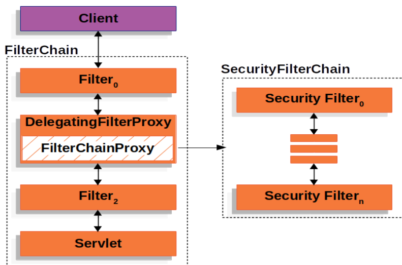
Рисунок 12 – SecurityFilterChain
