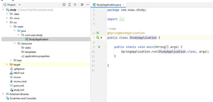
Рисунок 6 – Сгенерированный проект
