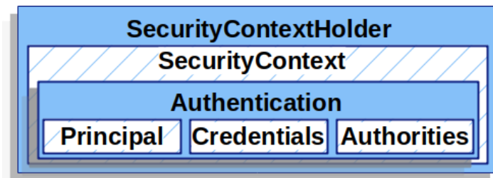
Рисунок 14 – SecurityContextHolder
