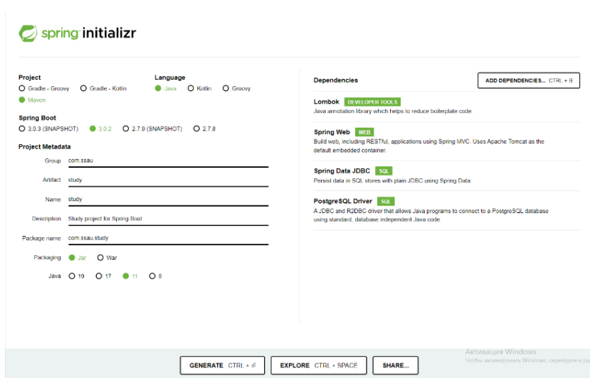
Рисунок 5 – Онлайн-инициализатор приложений
