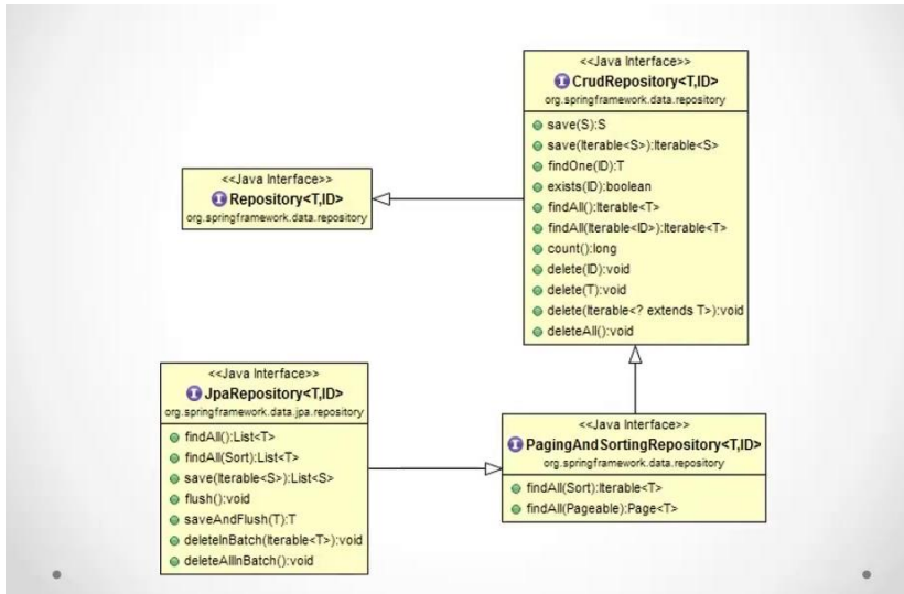
Рисунок 11 – Иерархия интерфейсов
