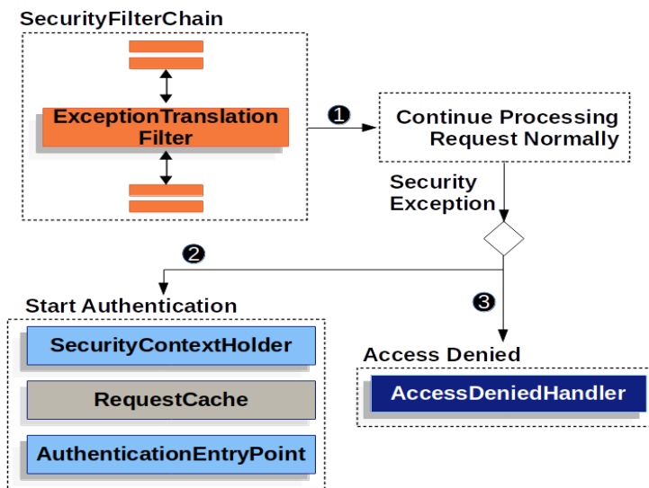
Рисунок 13 – Обработка исключений
