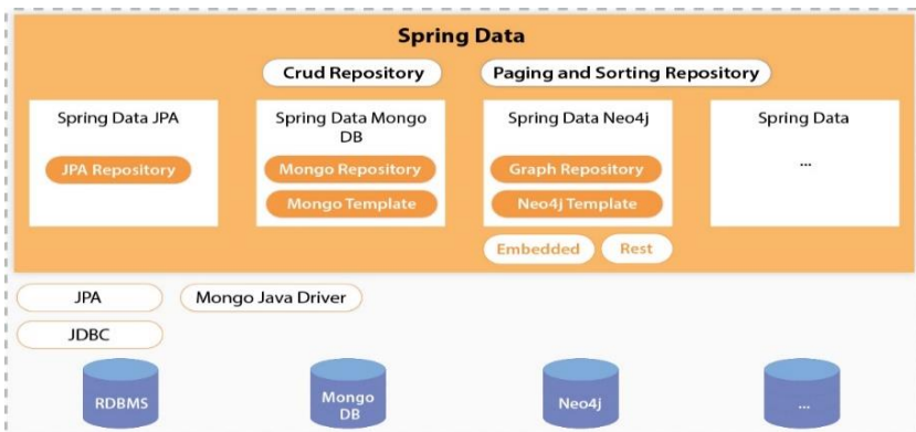
Рисунок 9 – Spring Data
