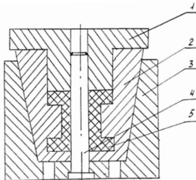
Рис. 4.9. Схема пресс-формы прямого прессования с двумя плоскостями разъема – вертикальной и горизонтальной: 1 – пуансон; 2 – матрица; 3 – обойма; 4 – знак; 5 – деталь
