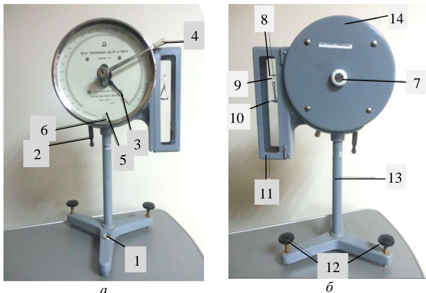
Рис. 2.2. Торсионные весы:
