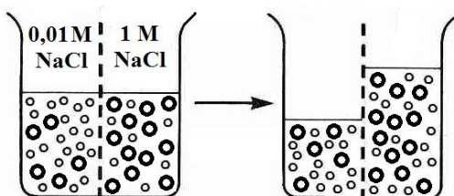
Рис. 1.2. Схема осмоса: крупные кружки – ионы Na + и Cl - ; мелкие кружки – молекулы воды
