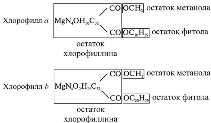
Рис. 3.1. Строение молекул хлорофиллов a и b
