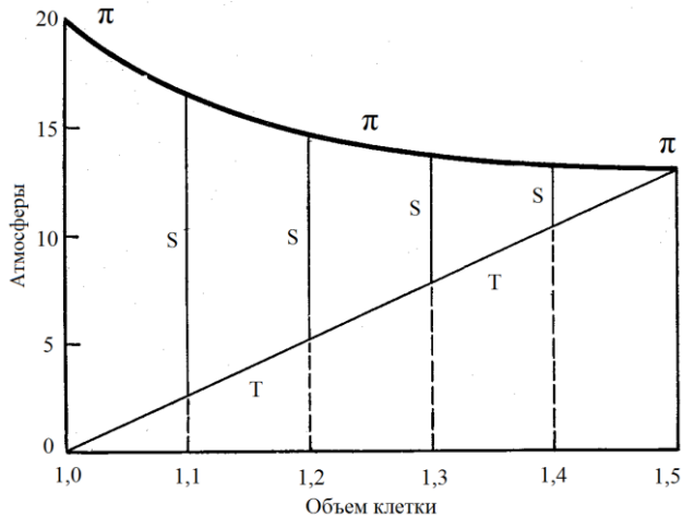
Рис. 1.6. Схема изменения осмотических величин в клетке в зависимости от ее насыщенности водой
