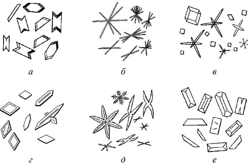
Рис. 5.2. Кристаллы гидротартрата калия (а), гипса (б), аммонийно-фосфорного молибдата (в), сульфата серебра (г), фосфорно-аммиачно-магнезиальной соли в случае быстрой (д) и медленной (е) кристаллизации
