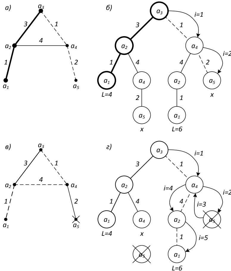
Рис. 1. Иллюстрация к возможности получения тупиковых решений в задаче поиска кратчайшего пути: а – исходный граф (жирным выделен искомый кратчайший путь между вершинами a_3 и a_1 , пунктиром показано тупиковое жадное решение); б – соответствующее комбинаторное дерево; в – жадное решение при запрете посещения тупиковой вершины a_5 ; г – порядок обхода узлов комбинаторного дерева с учетом возврата из тупиковой вершины a_5
