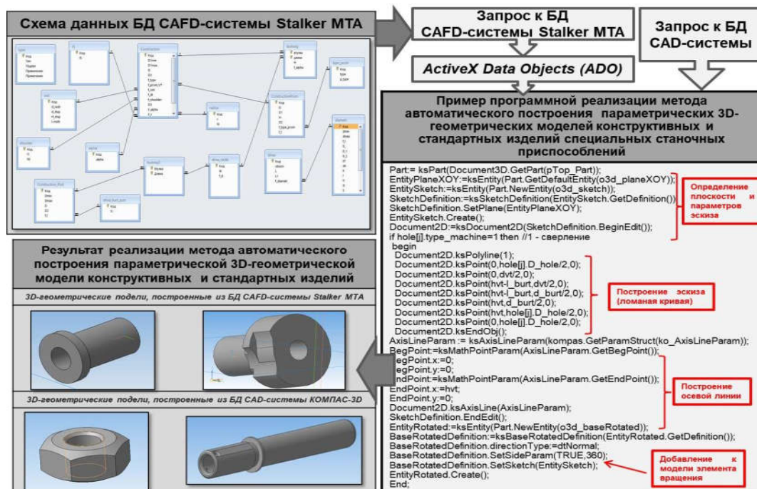
Рисунок 1 – Фрагмент схемы данных БД системы CAFD Stalker MTA
