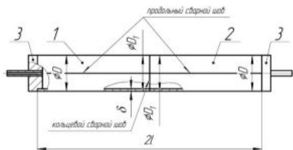
Рис. 1. Эскиз экспериментального образца: 1 – цилиндрическая оболочка из стали 12X18H10T; 2 – цилиндрическая оболочка из стали 321; 3 – колпак со штурцером
