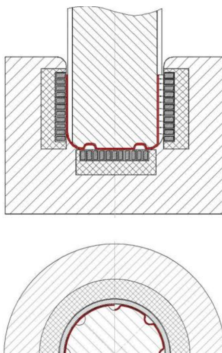
Рис. 2. Комбинированная технология вытяжка-формовка
