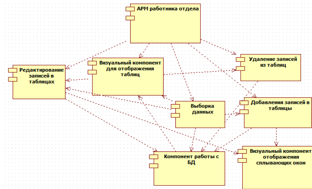
Рис. 1. Диаграмма компонентов
