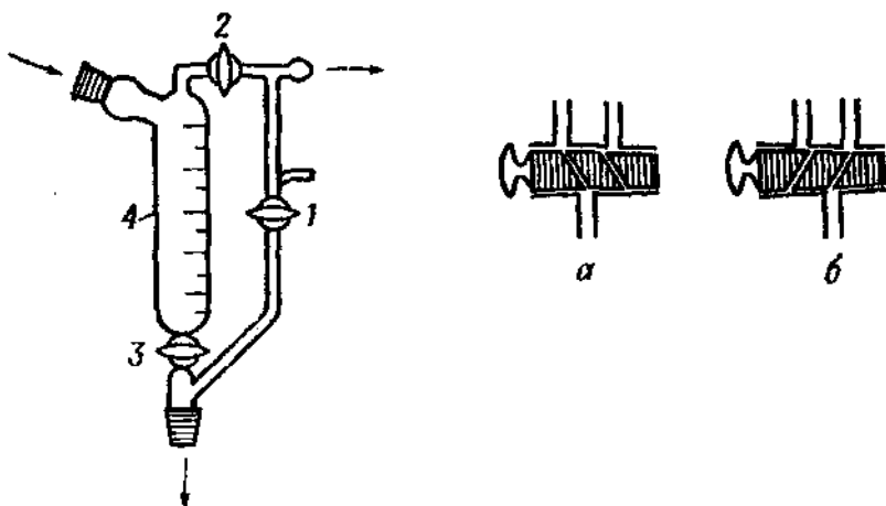
Рис. 11. Форштос Аншютца – Тиле.
