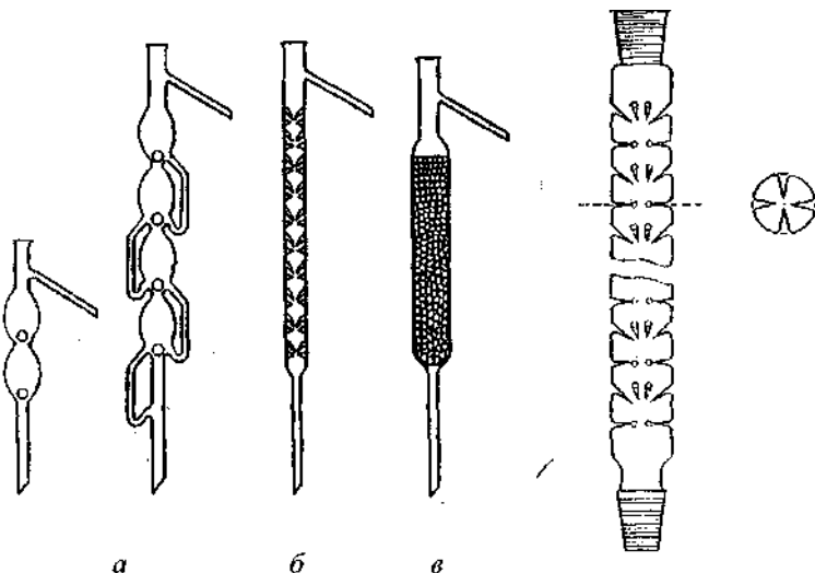
Рис. 13. Дефлегматоры:
