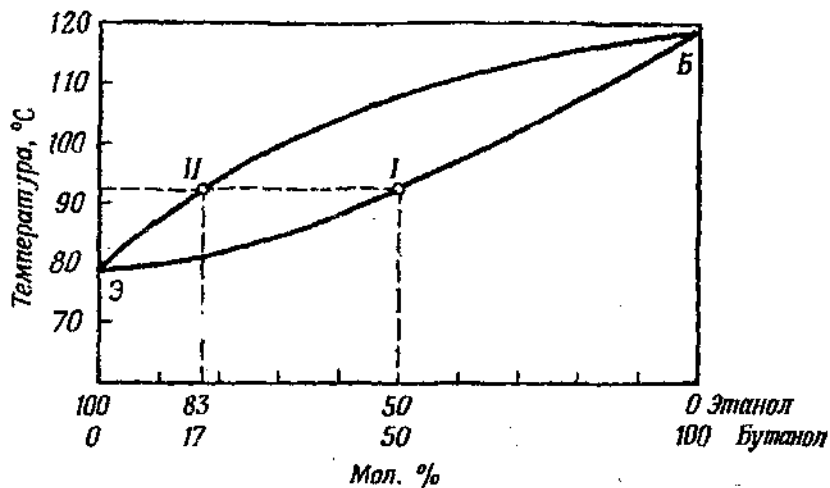
Рис. 12. Диаграмма кипения смеси этанол – бутанол-1.
