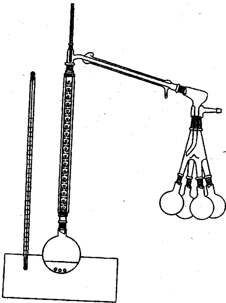
Рис. 15. Установка для перегонки бинарной смеси.
