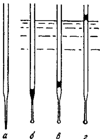
Рис. 4. Определение температуры кипения по Эмиху.
