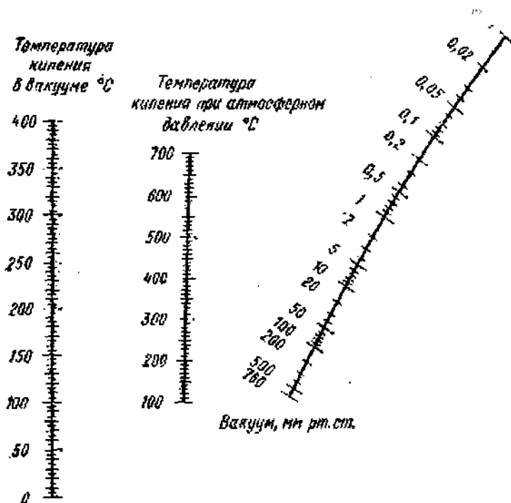
Рис. 8. Номограмма для определения температуры кипения в вакууме.
