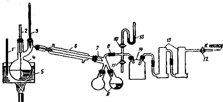
Рис. 9. Установка для вакуумной перегонки:
