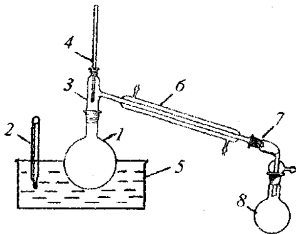
Рис. 5. Прибор для простой перегонки, собранный на шлифах.
