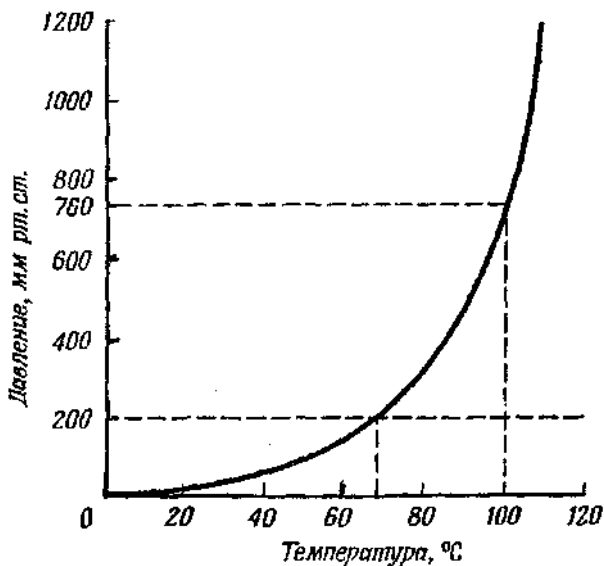
Рис. 2. Кривая давления водяного пара.
