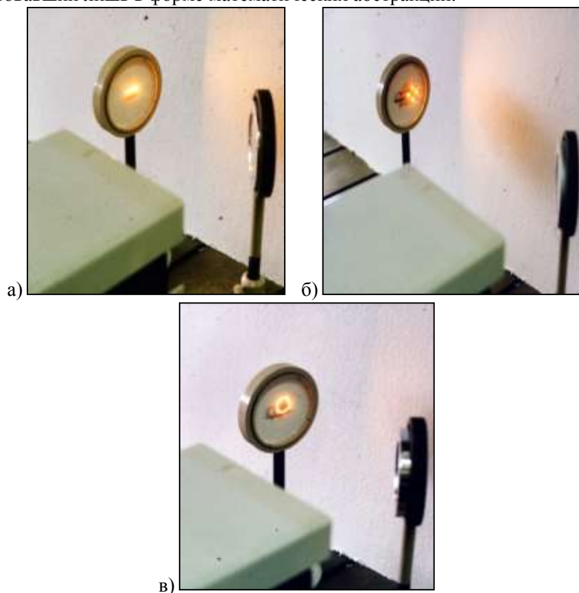
Рисунок 2. Распределение интенсивности излучения \text{CO}_2 - лазера, сформированные фокусаторами: в поперечный отрезок (а), в четыре точки (б) и в кольцо (в).
