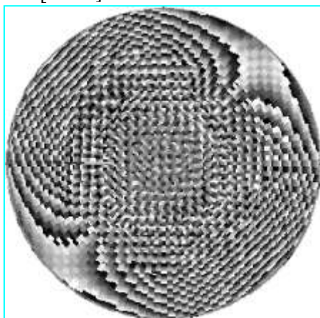
Рисунок 4. Фотошаблон для многоканального модана.
