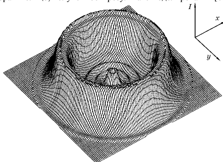
Рисунок 5. Расчетное распределение интенсивности в фокальной плоскости фокусатора в кольцо.
