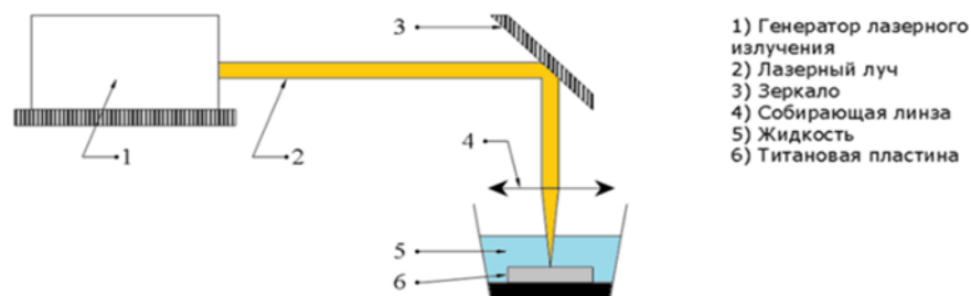
Рис 1 – Экспериментальная установка
